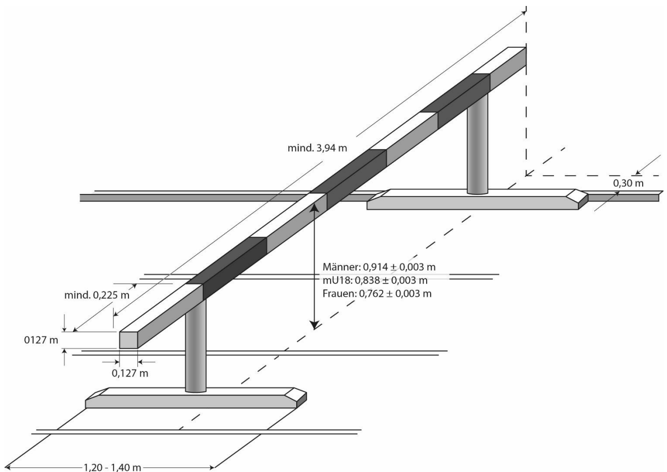
Zeichnung 6: Hindernisabmessungen
