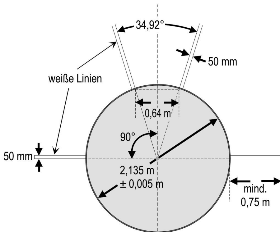
Zeichnung 20: Hammerwurfkreis
