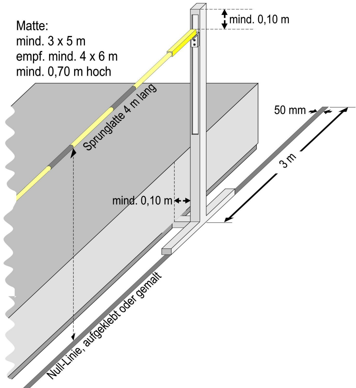
Zeichnung 10: Hochsprunganlage
