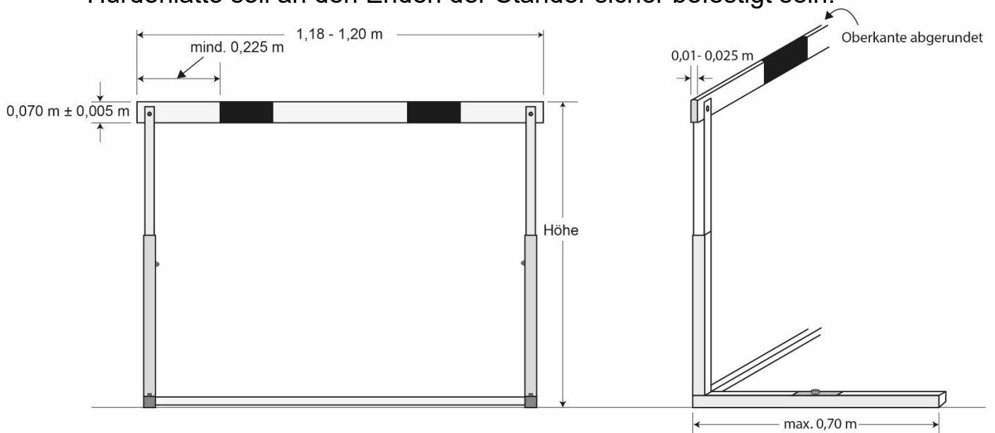
Zeichnung 4: Hürdenabmessungen
