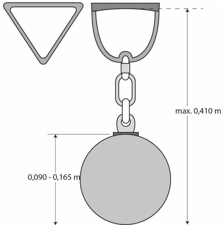
Zeichnung 31: Wurfgewicht
